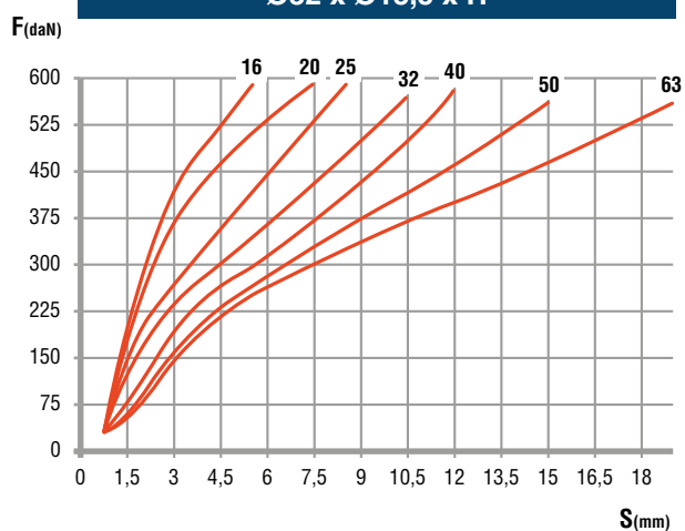
Ø32 x Ø13,5 x H
