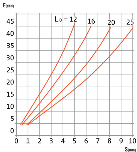
Ø25 x Ø10,5 x H
