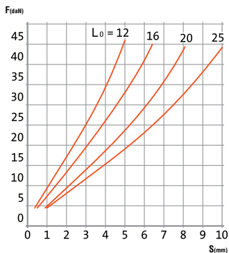
Ø25 x Ø10,5 x H
