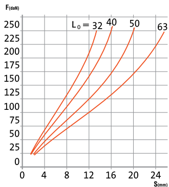
Ø32 x Ø13,5 x H
